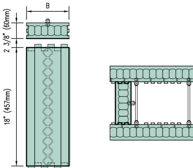
END CAP
